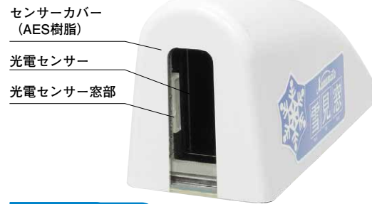
降雪センサーYMS3形
