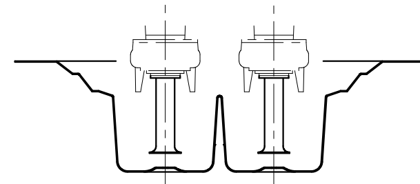
ベルマウス詳細図
