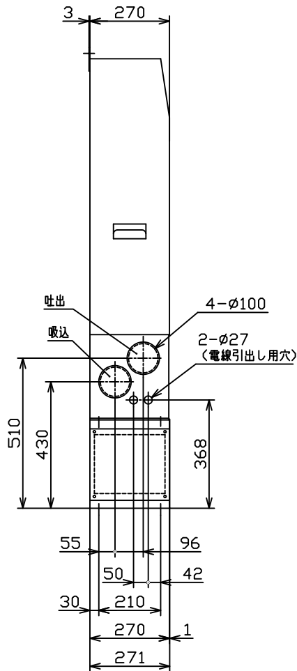
断面AA(本体下部詳細)
