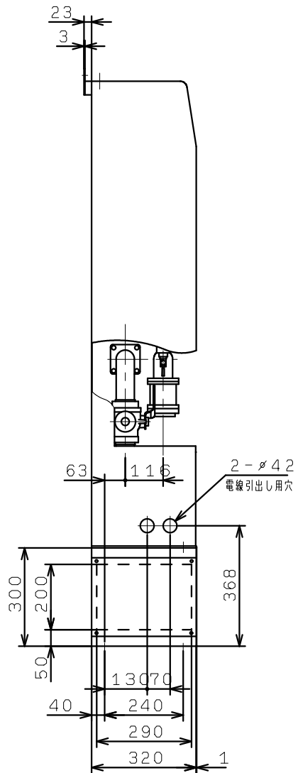
矢視A (本体下部詳細)
