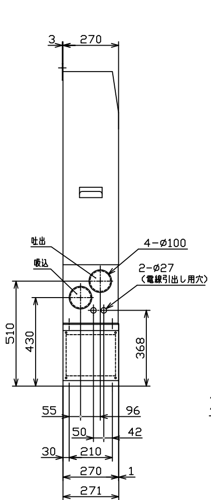
断面AA(本体下部詳細)
