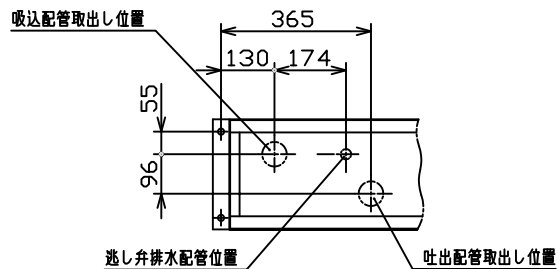
断面AA(本体下部詳細)
