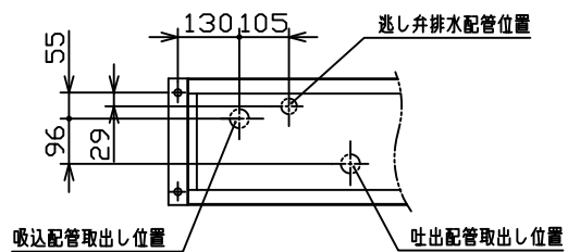
断面AA(本体下部詳細)
