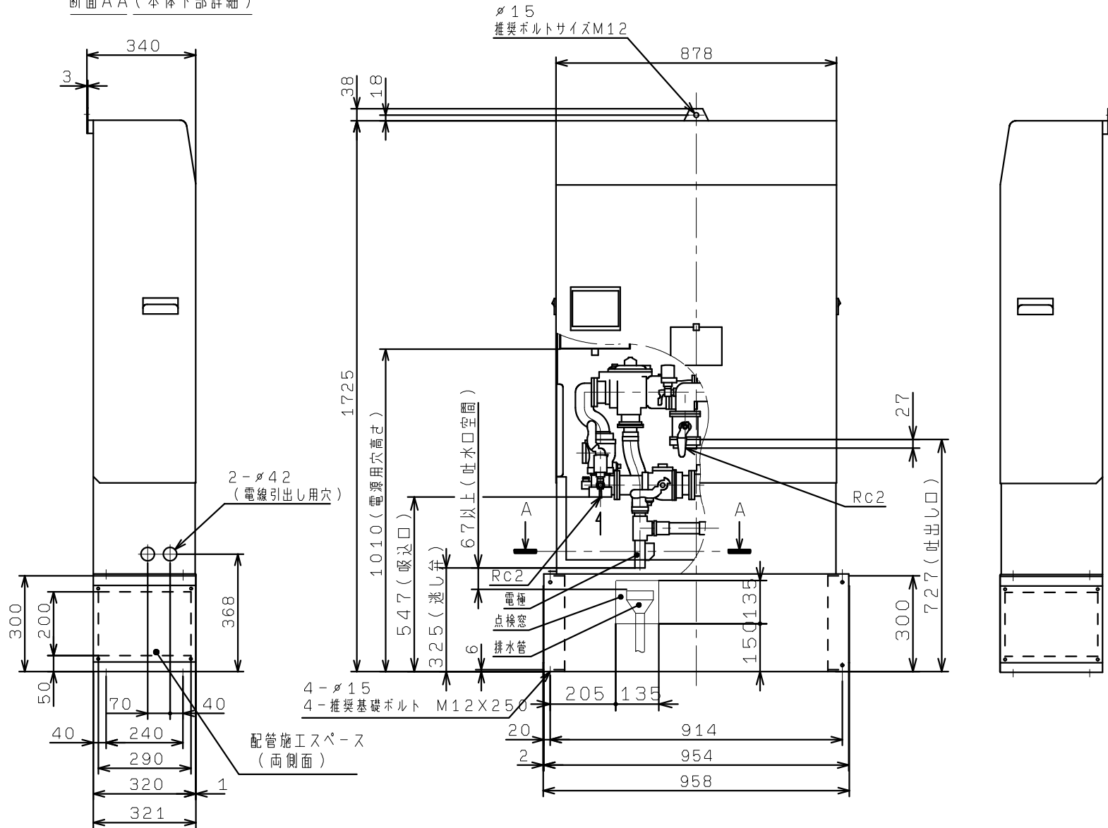
断面A A (本体下部詳細)
