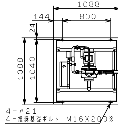
断面A-A
