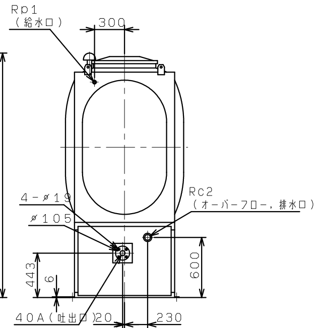
断面A-A
