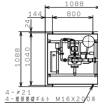
断面A-A
