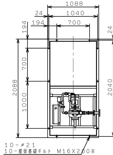
断面A-A
