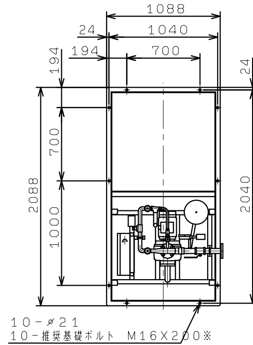
断面A-A
