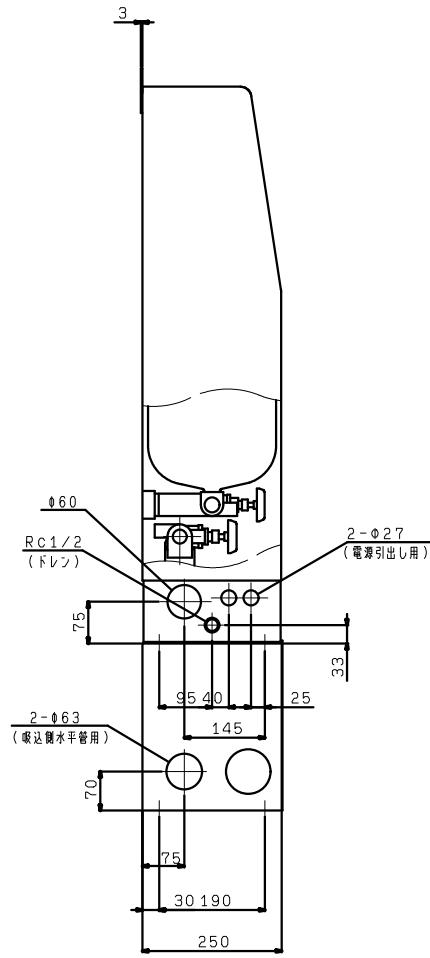
矢視A (本体下部詳細)
