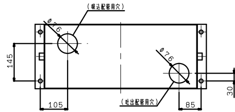
矢視A (本体下部詳細)
