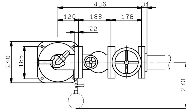
チェック弁/スルース弁付
