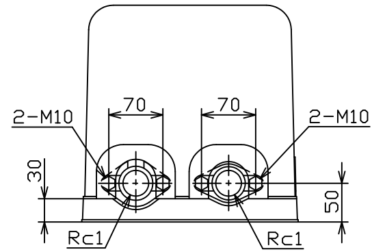
矢視A
