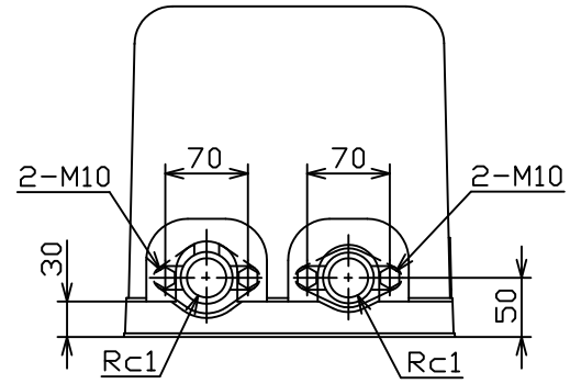
矢視A
