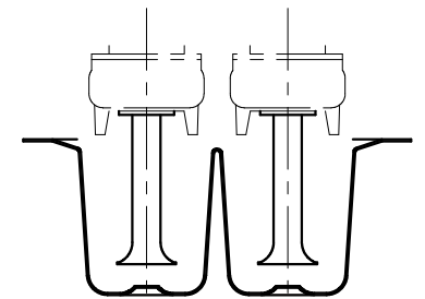
ベルマウス詳細図
