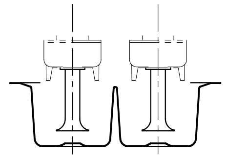
ベルマウス詳細図
