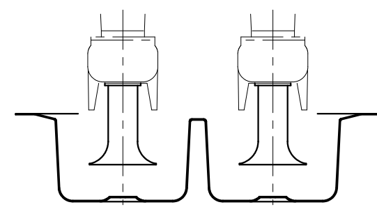
ベルマウス詳細図
