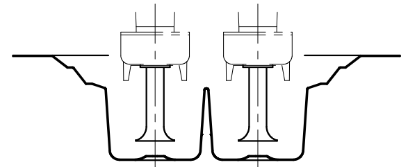
ベルマウス詳細図
