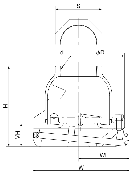
VFST2形 (ねじ込み式)
