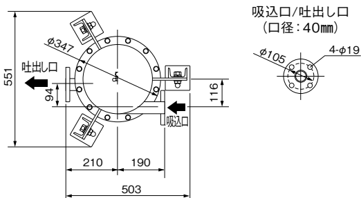
矢視 A
