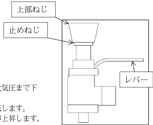
<図-8>：圧力調整弁
