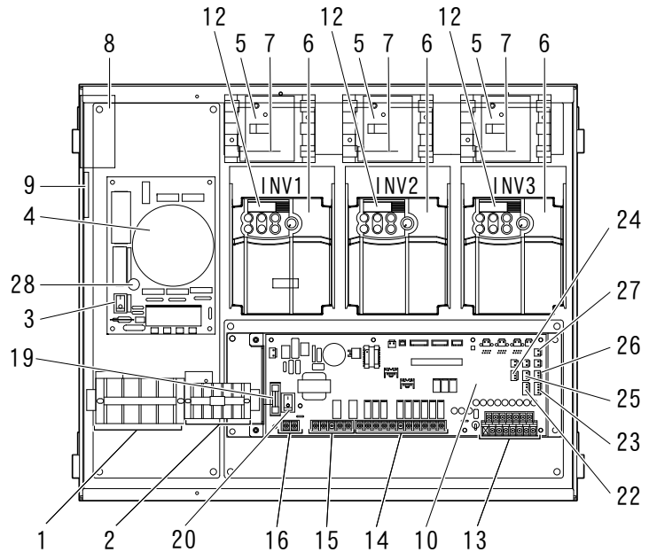
<制御盤内部>
