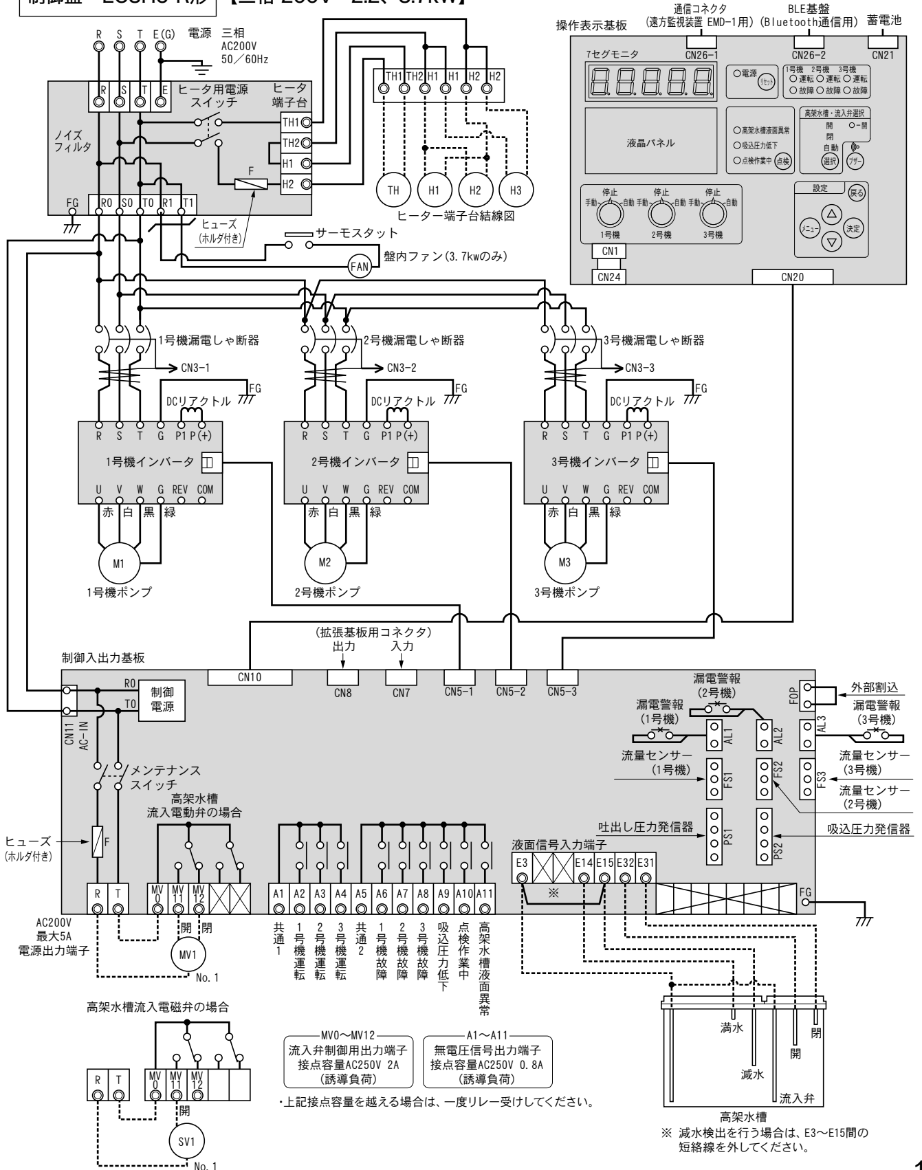
制御盤 - ECSH5-R形 【三相 200V 2.2、3.7kW】
