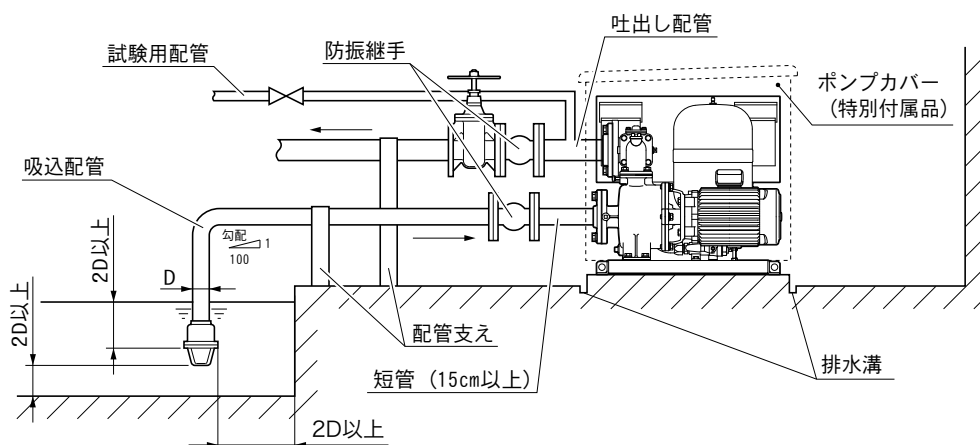
[地下水槽からの吸上げにて使用する場合]
